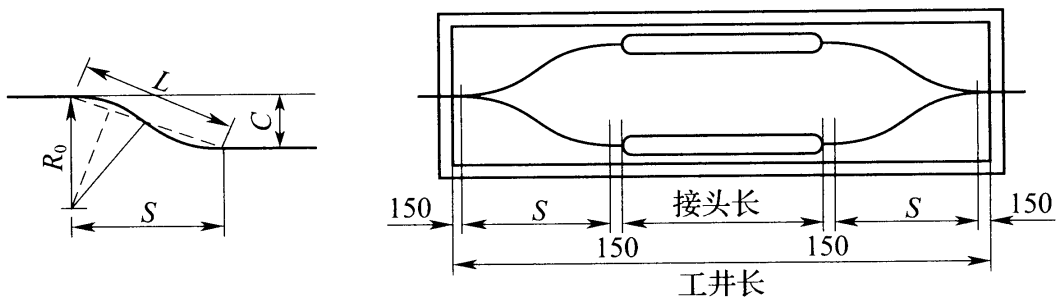
(b) 工井顶视图
