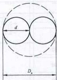
图 1 1×2 结构钢绞线外形示意图
