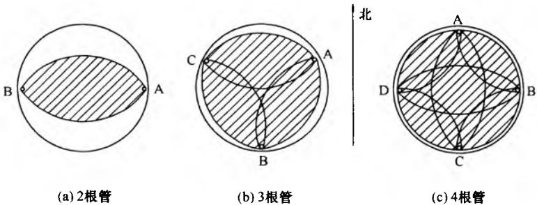
图 10.3.2 声测管布置示意图
