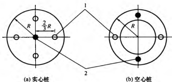
图1 传感器安装点、激振（锤击）点布置示意图
