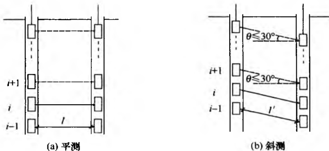
图 10.4.2 平测、斜测示意图
