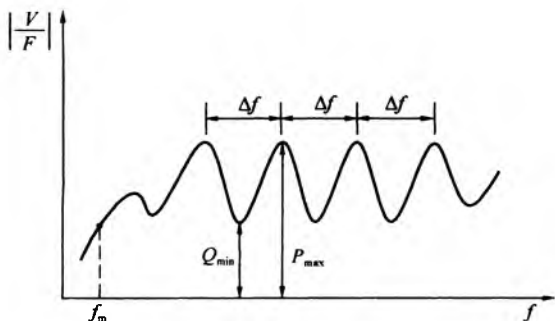
图6 均匀完整桩的速度导纳曲线图
