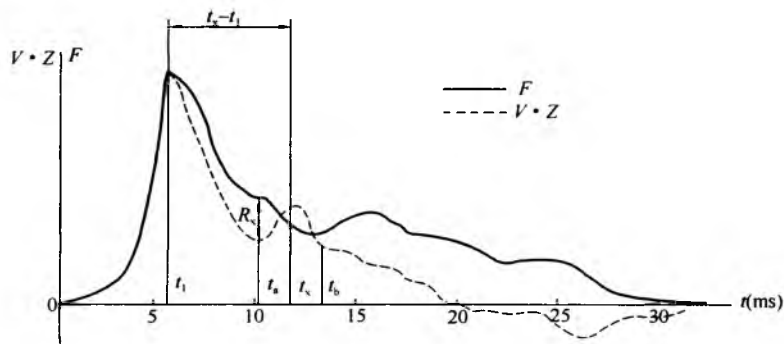
图 9.4.11 桩身完整性系数计算
