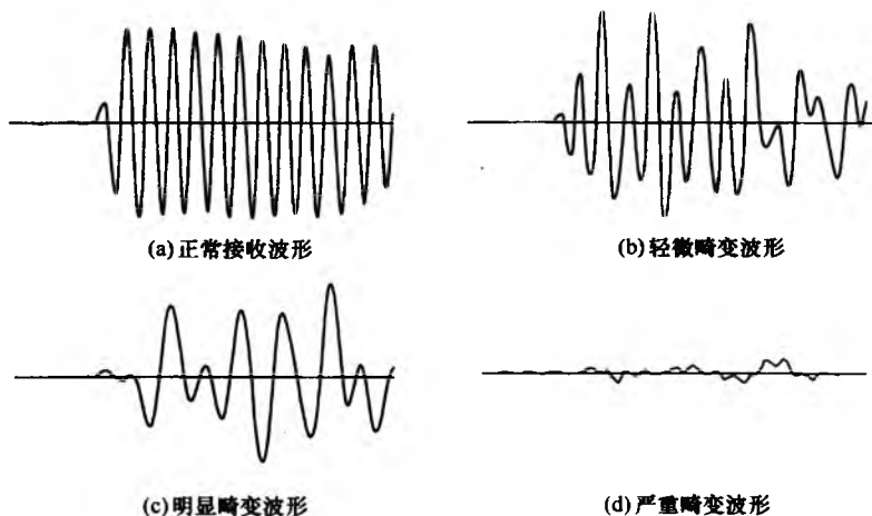
图 13 接收波形畸变程度示意
