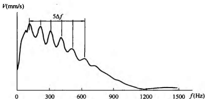
图 3 完整桩典型速度幅频信号特征
