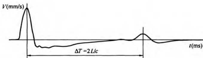
图 2 完整桩典型时域信号特征
