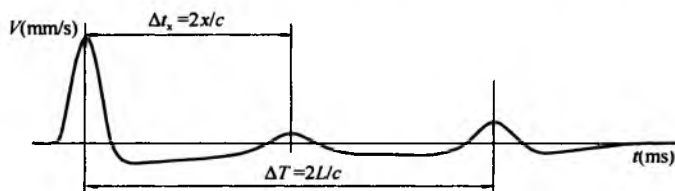
图 4 缺陷桩典型时域信号特征
