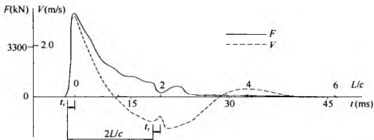
图 9.4.3 桩身波速的确定
