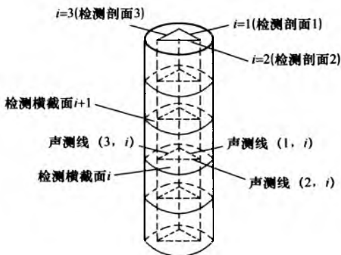
图 10 检测剖面、声测线、检测横截面编组和编号示意图
