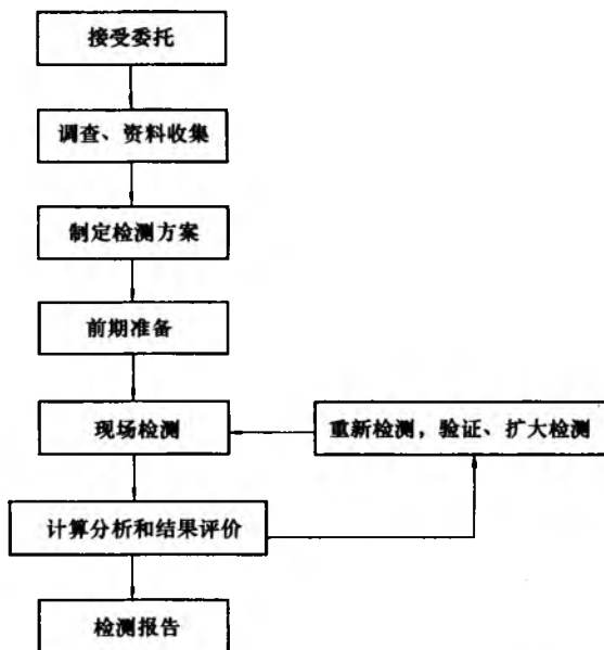
图 3.2.1 检测工作程序框图
