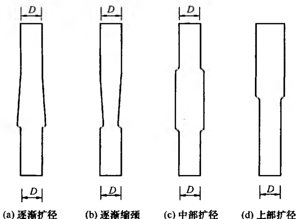
图7 混凝土灌注桩截面（阻抗）变化示意图
