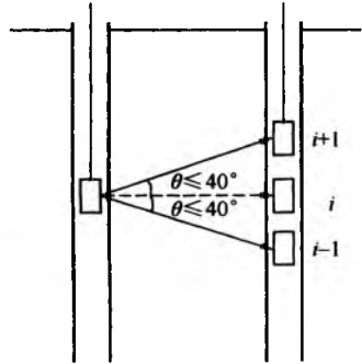
图 10.4.3 扇形扫测示意图
