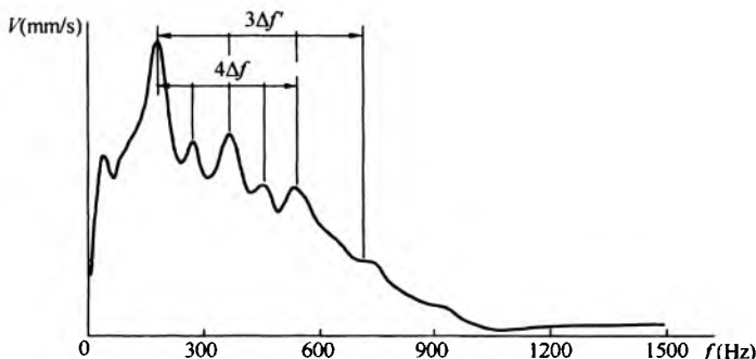
图5 缺陷桩典型速度幅频信号特征
