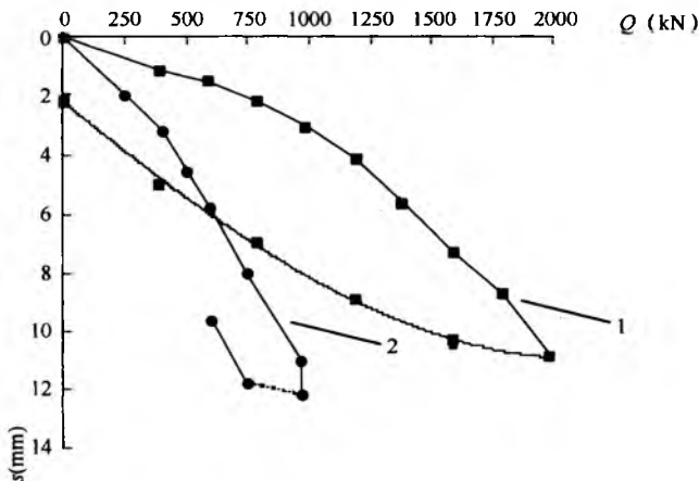
图9 静载和动载模拟的 Q-s 曲线
