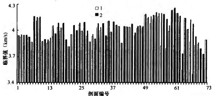
图 11 21 根桩 72 个检测剖面双剔法与单剔法的 异常判断概率统计值比较 1—单边剔除法；2—双边剔除法
