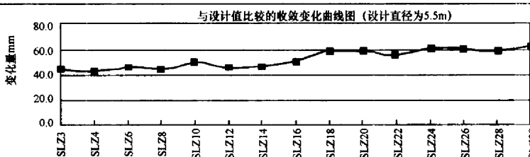
图 41 固定测线法收敛监测报表和变化曲线图
