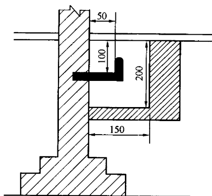
图 32 窞井式标志
