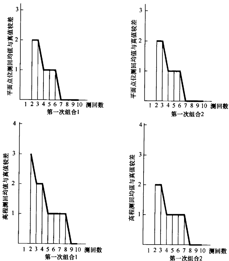
图8 激光扫描测量平面位置及高程较差与测回数关系
