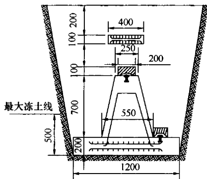
图 14 混凝土基本水准标石 (单位: mm)
