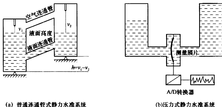
图1 连通管式与压力式静力水准系统原理图
