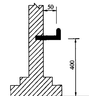
图 18 铸铁或不锈钢墙体明标水准标志 (单位: mm)
