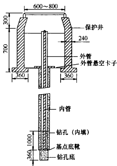
图 13 深埋钢管水准基点标石 (单位: mm)
