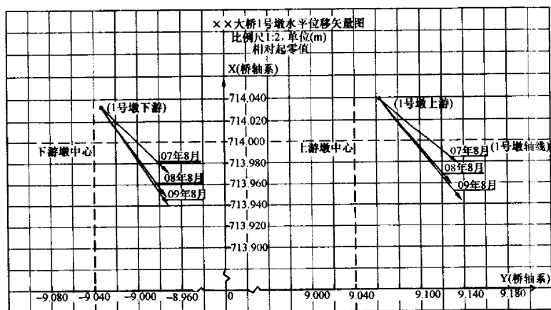
图 37 水平位移图
