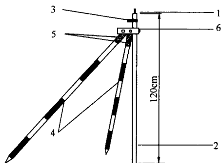
图5 架设棱镜组的三脚架
