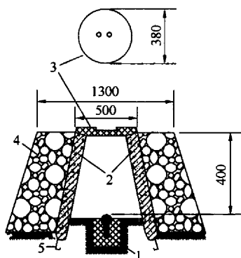
图 11 基岩水准基点标石 (单位: mm)
