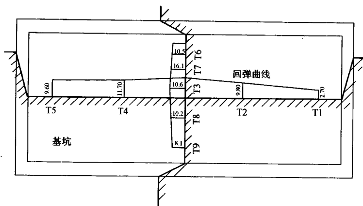
图31 基坑回弹监测点位布置图及回弹纵、横断面图
