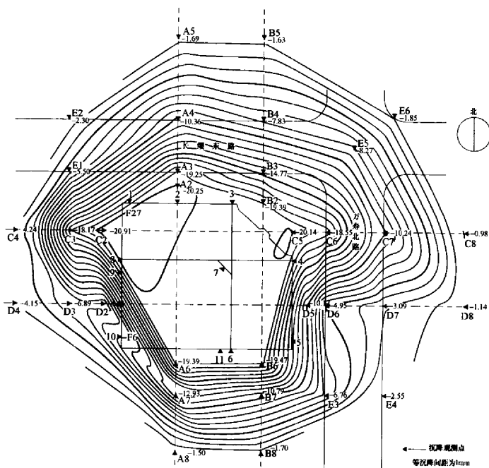
图 23 场地地面等沉降曲线
