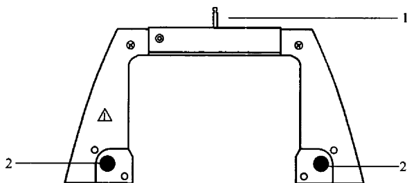
图6 用于安装棱镜组的全站仪提把 1—与棱镜组配套的连接杆；2—提把开关
