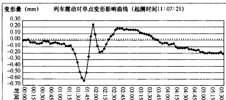
图 3 静力水准典型液面振荡曲线
