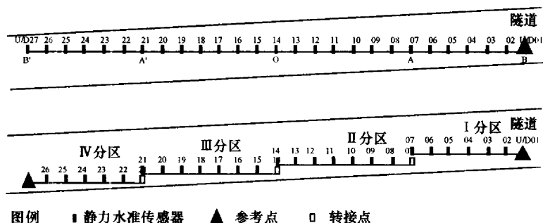
图2 静力水准线路分组安装示意图
