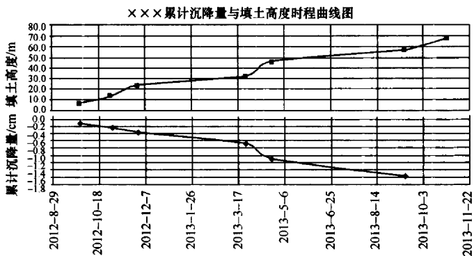
图 27 各土层沉降量-填土高度时程曲线
