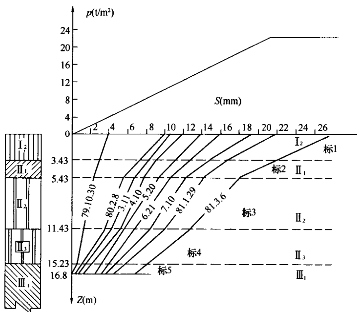
图 26 各土层荷载-沉降-深度曲线
