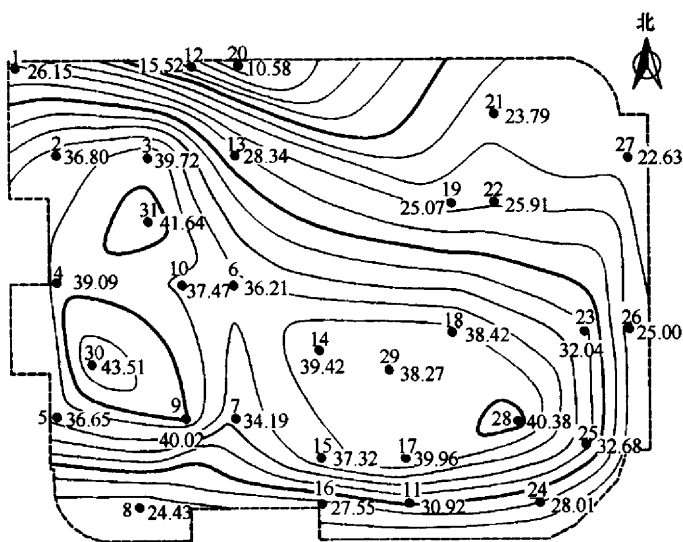
图 36 等沉降曲线
