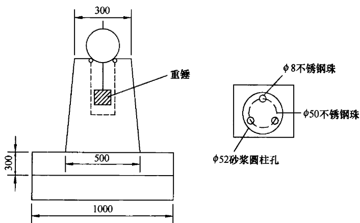
图 21 重力平衡球式照准标志 (单位: mm)
