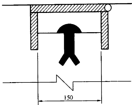
图 33 盒式标志
